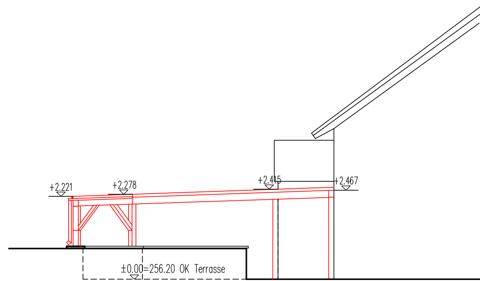
Seitenansicht/Ost
