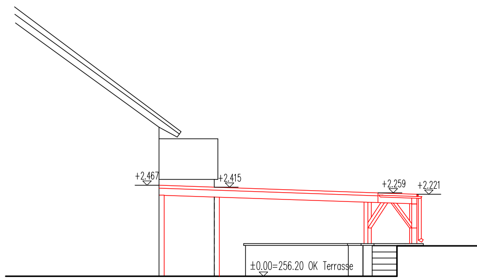
Seitenansicht/West
