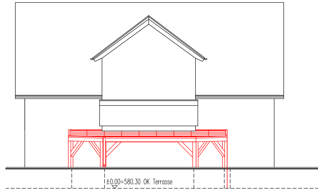
Vorderansicht/Süd
